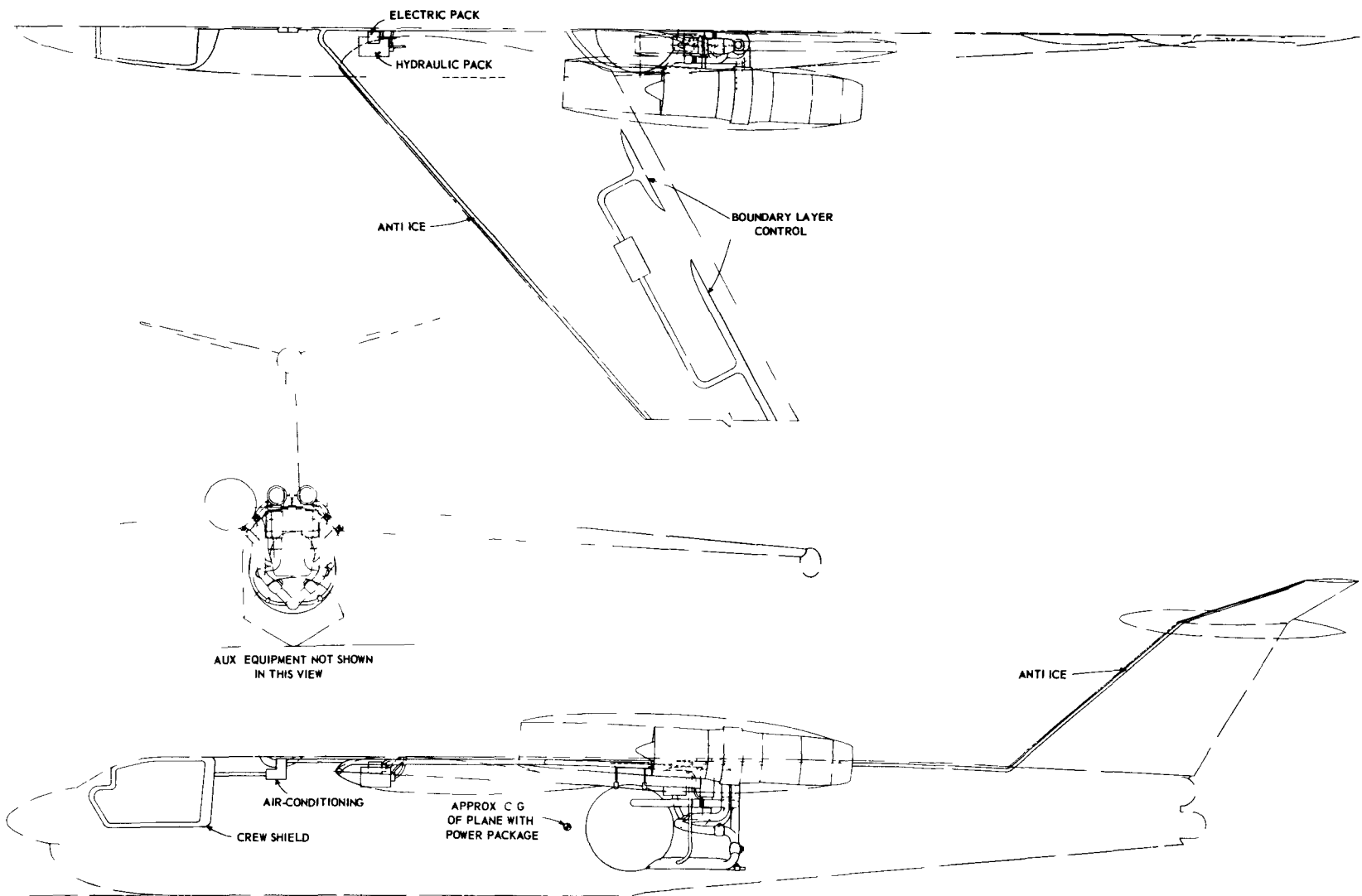
Fig. 2.9 – CCR power-plant installation
